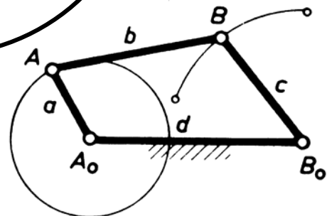
Kurbelschwingen
