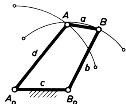
Doppelschwinge
