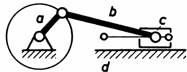
Schubkurbel
