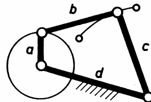
Kurbelschwinge
