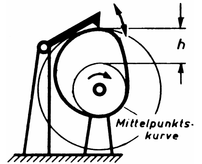
Schwinghebel
