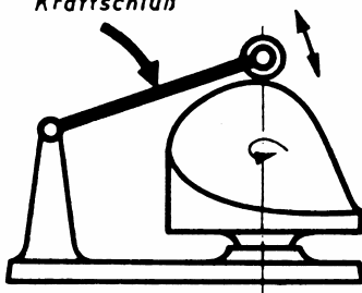
Kraftschluß
