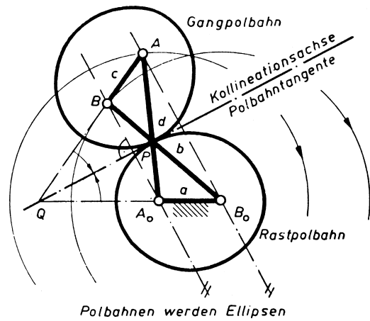
Antiparallelkurbeln gegenläufig
