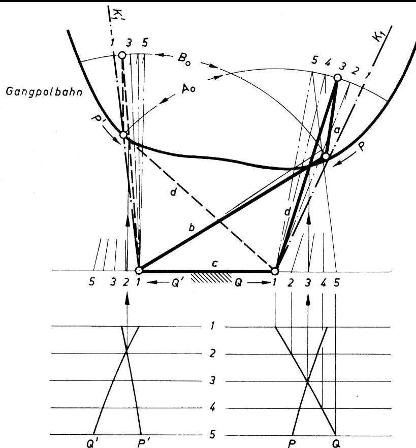
Ermittlung der Getriebelagen für k \perp c
