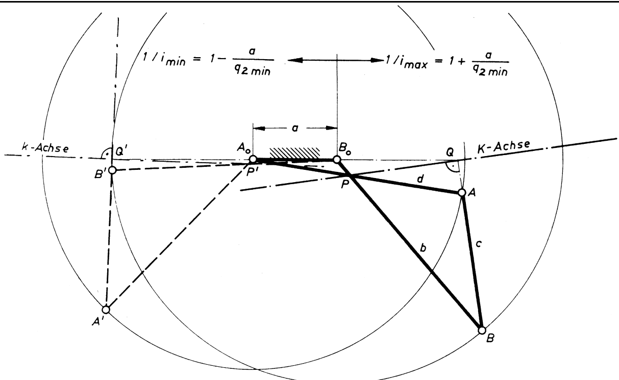
Ermittlung der Getriebelagen für k \perp c
