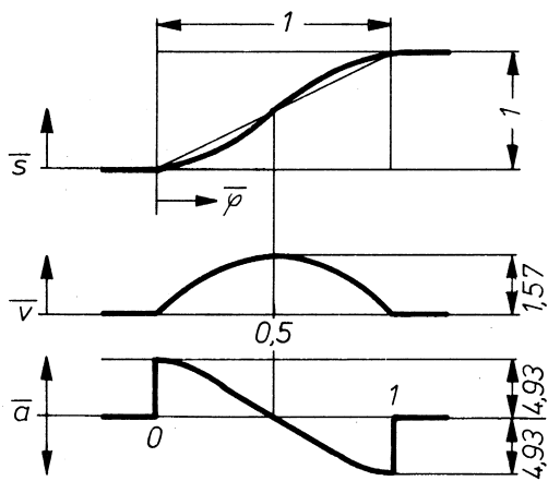
Einfache Sinuide
