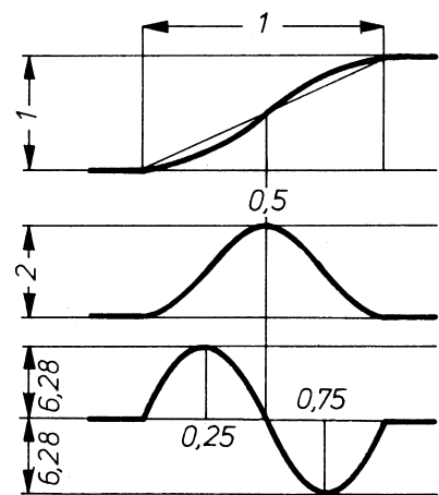
Geneigte Sinuslinie
