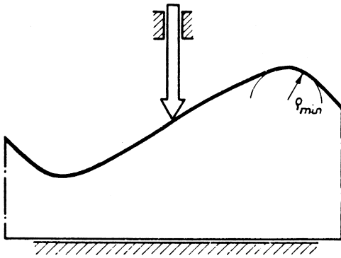
a Kurvenflanke = Mittelpunktsbahn
