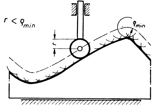
b Kurvenflanke ist Äquidistante
